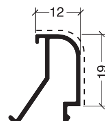
ADR 914 Contravidrio curvo 12 mm 0,209 kg/m
