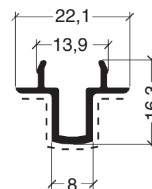
ADR 1651 Encuentro central 4 hojas 0,180 kg/m
