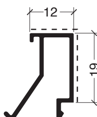
ADR 913 Contravidrio recto 12 mm 0,216 kg/m
