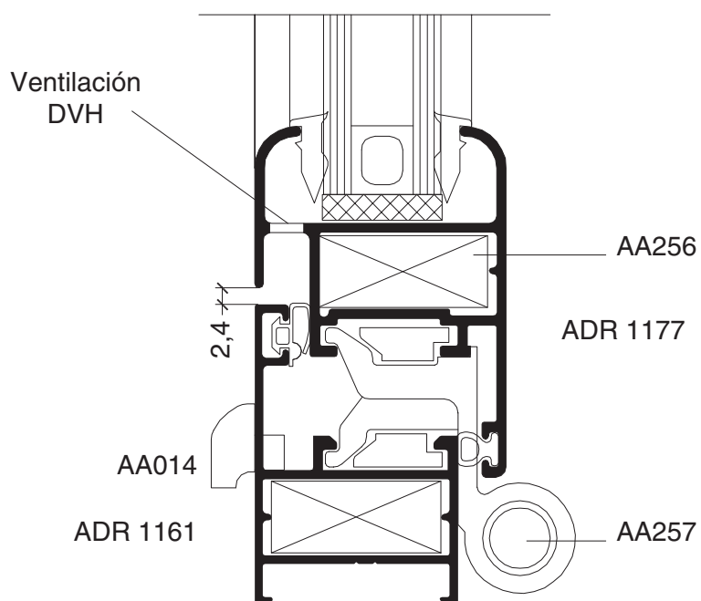
Secciones (Escala 1:1)
