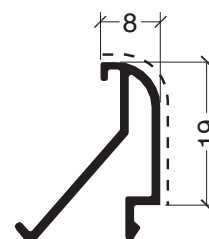
ADR 911 Contravidrio curvo 8 mm 0,203 kg/m
